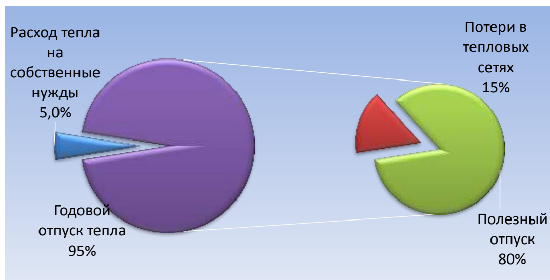
Рисунок 1.6.1.2 Годовой отпуск тепла от котельной №14.
