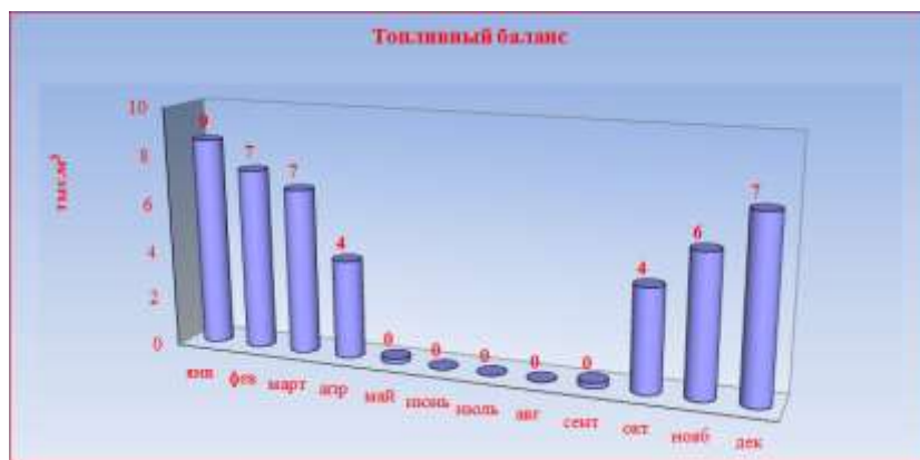
Рисунок 8.1.1 Перспективный расход топлива для котельной №14
