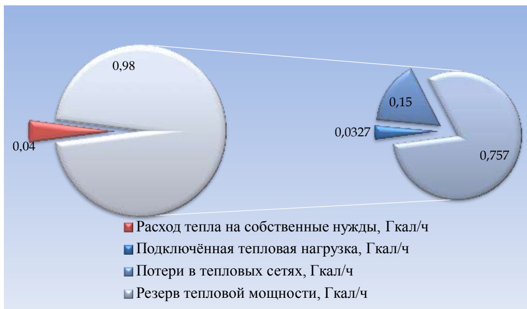
Рисунок 1.6.2.1 Тепловой баланс котельной №15
