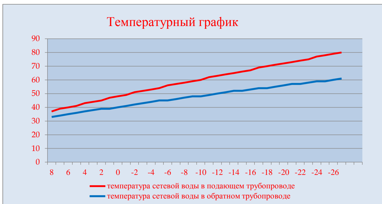
Рисунок 1.2.1. Рисунок температурного графика работы котельных
