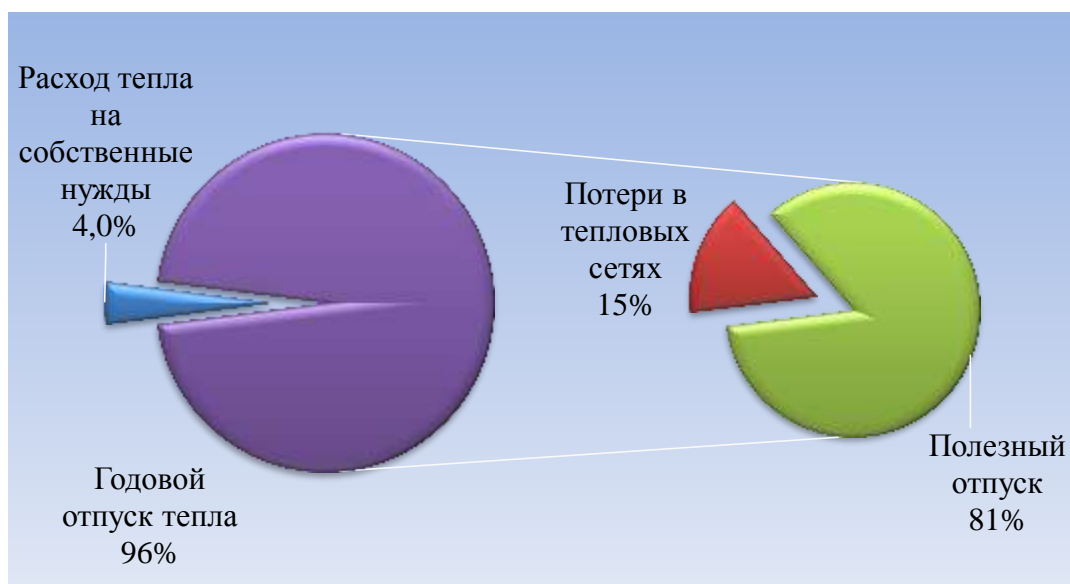
Рисунок 1.6.2.2 Годовой отпуск тепла от котельной №15.
